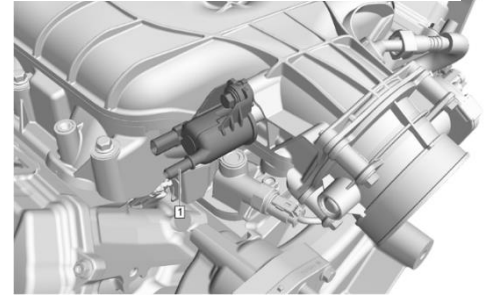
ORIFICE D'ÉMISSION DE VAPEURS DE CARBURANT
