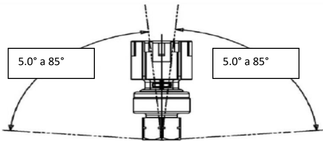
ORIENTACIÓN DE MONTAJE PERMISIBLE EN CUALQUIER DIRECCIÓN RELATIVA A LA POSICIÓN VERTICAL
